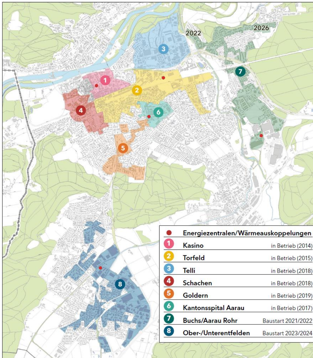
Übersicht der bestehenden und geplanten Energieverbunde von Eniwa.
